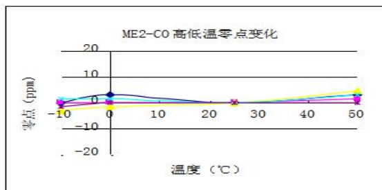
探头高低温零点变化图
