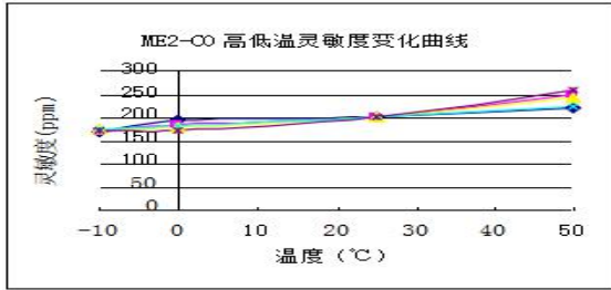
探头干低温灵敏度变化曲线
